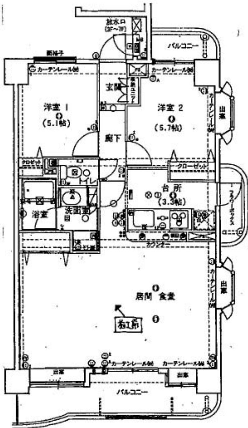
既存平面図
